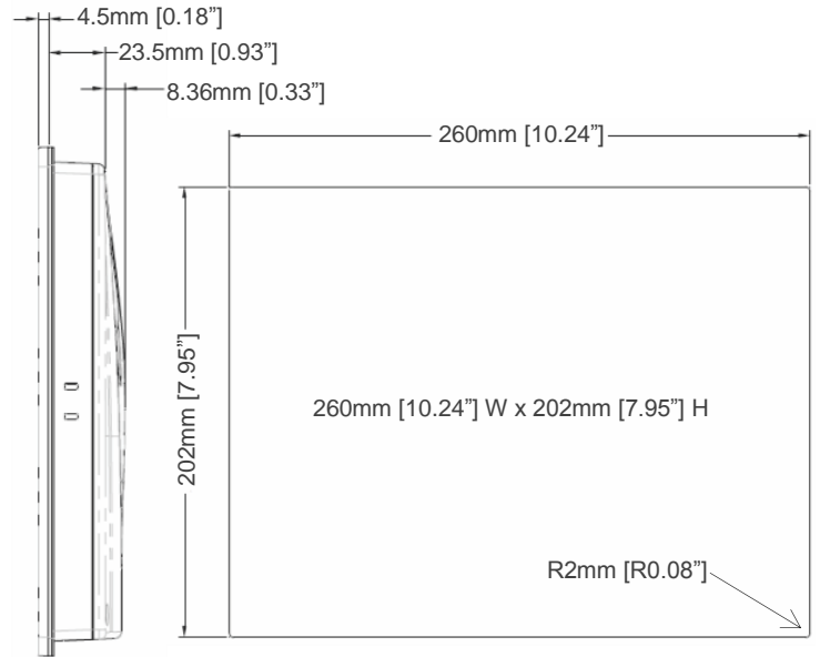
Cutout Dimensions
