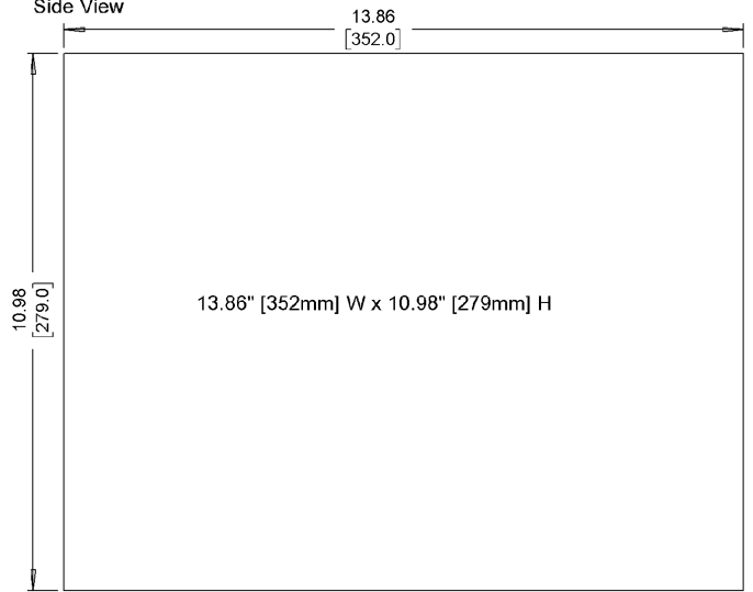
Cutout Dimensions
